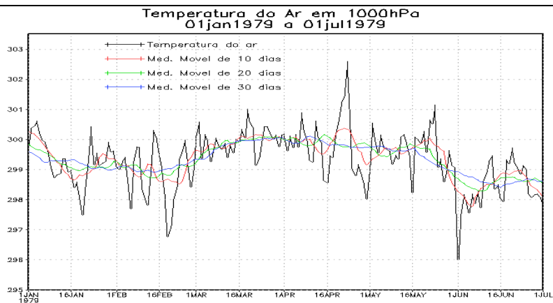
Figura 37 – Gráfico de Média Móvel.
